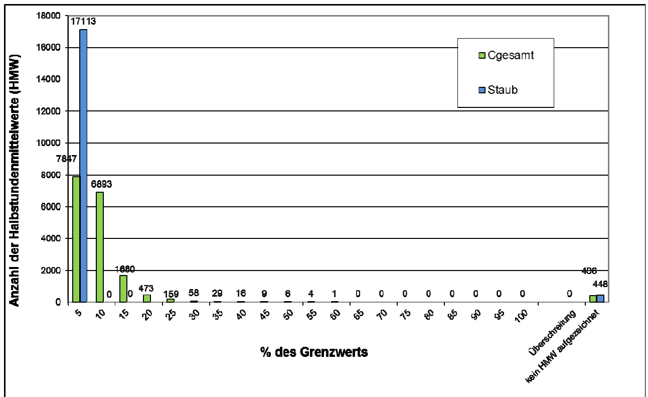
Diagramm 1: Klassenhäufigkeitsverteilung der Halbstundenmittelwerte 2016
